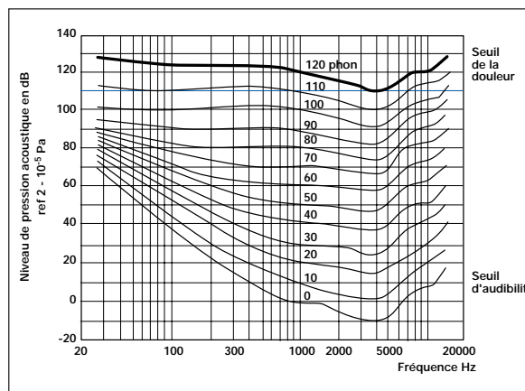
Diagramme Fletcher - Munson Courbes isophoniques
