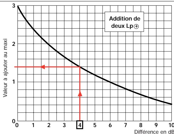
Fig. 5 : addition de 2 niveaux sonores
