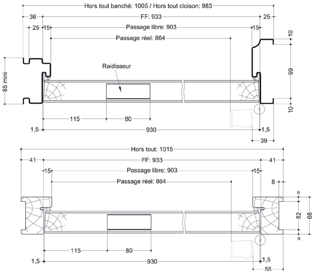
BP PHONIBLOC AR grande largeur avec raidisseur
