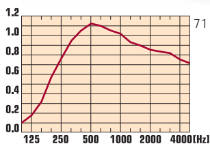
delta avec 40 mm Isolation h 59 mm
