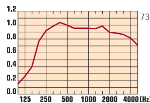
delta avec 40 mm Isolation h 159 mm
