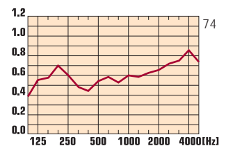
delta avec 40 mm Isolation h 439 mm
