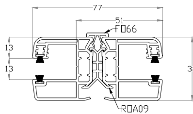
COULISSE DOUBLE R009 + R0A09 + F066
