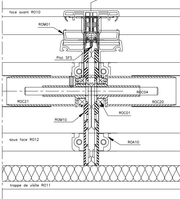
Une seule manoeuvre en extrémité
