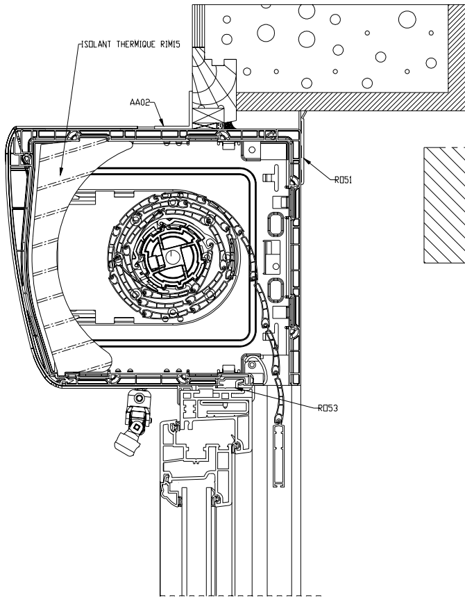
CVI EN REHABILITATION
