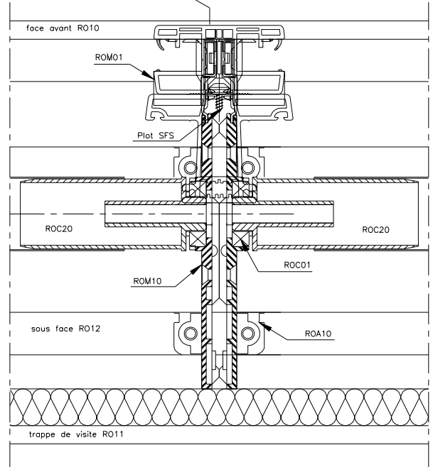
Deux manoeuvres en extrémité
