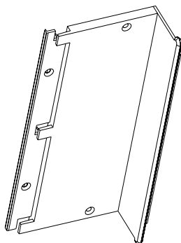
ENSEMBLE EMBOUS CVR 2100 REHA ROM60C
