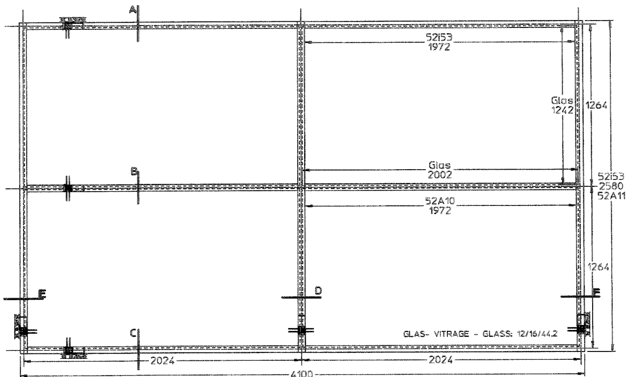
Snede/Coupe/Cut A
