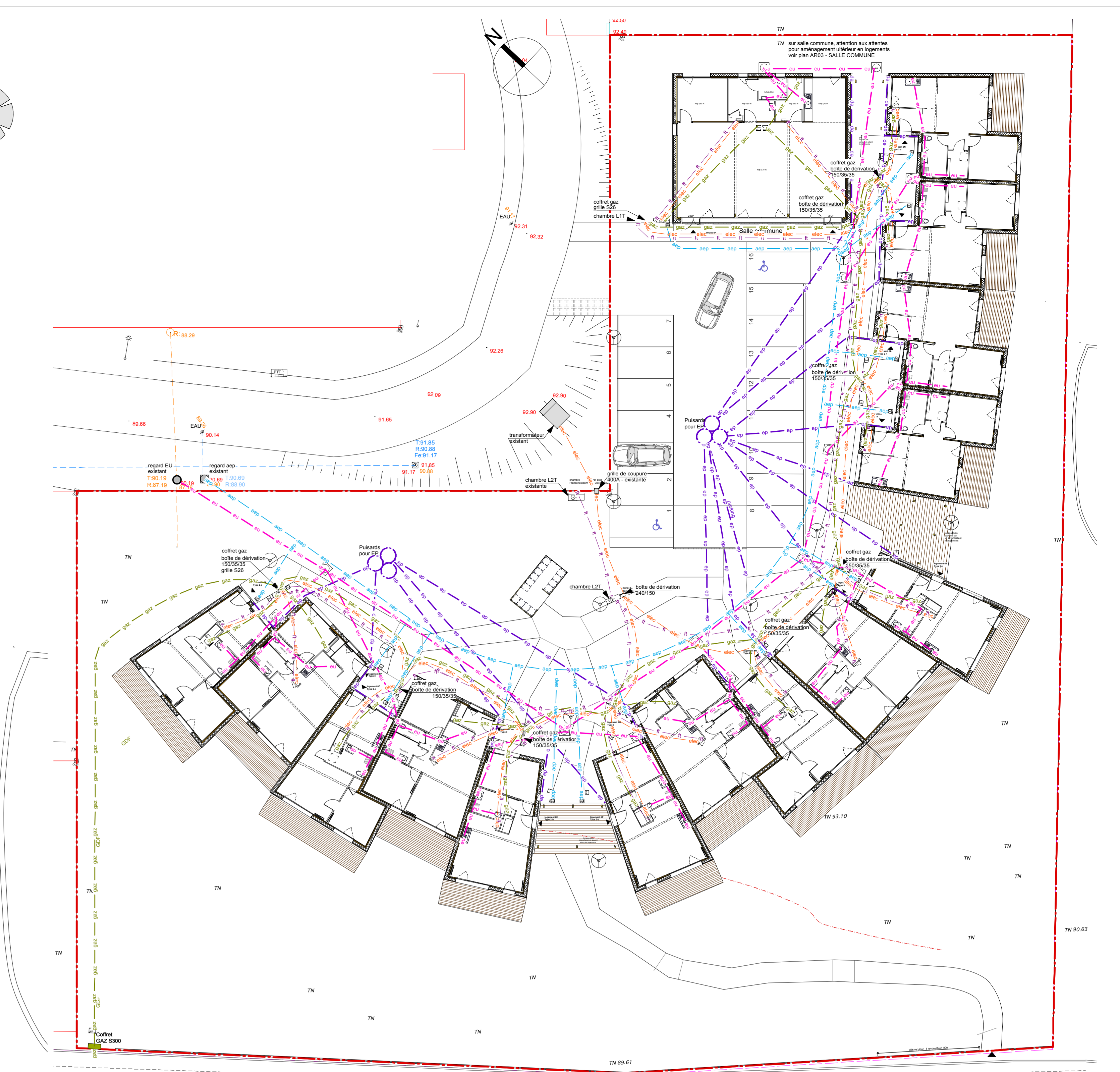
plan des réseaux - échelle 1/200
