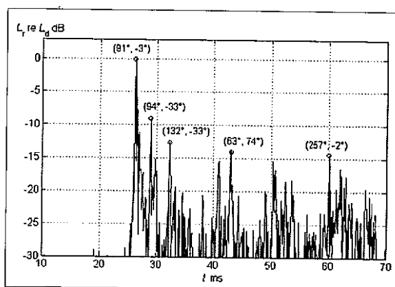
Fig. 10 : Echogramme spatial relevé sur la scène de l'auditorium. Le couple (azimut, élévation) de chaque contribution acoustique identifiée est indiqué
