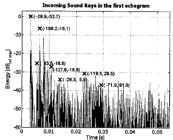
Fig. 7 : Échogramme de la salle test (rouge : le son direct, bleu : réflexions)
