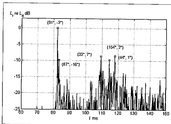
Fig. 12 : Relevé d'échogramme spatial dans la cathédrale avec l'assistance électroacoustique enclenchée
