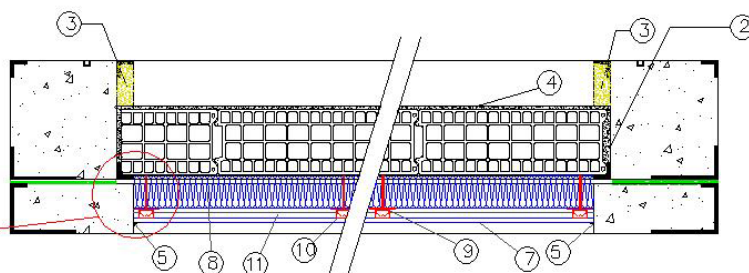
COUPE HORIZONTALE
