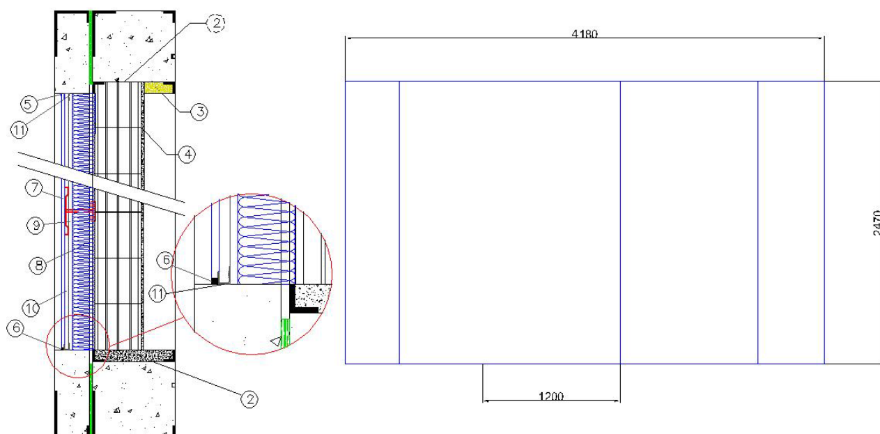
COUPE VERTICALE
