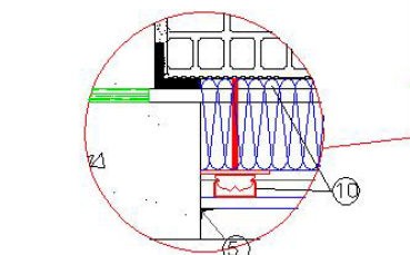
COUPE VERTICALE
