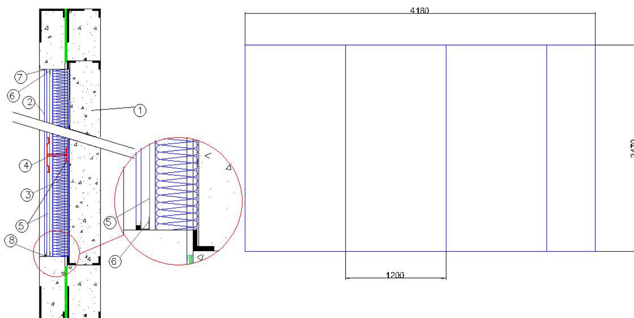
COUPE VERTICALE
