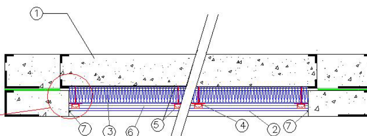
COUPE HORIZONTALE
