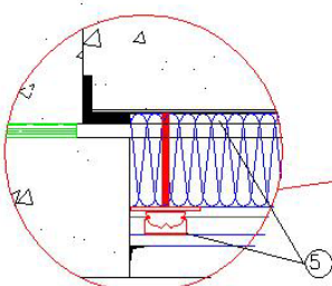
COUPE VERTICALE
