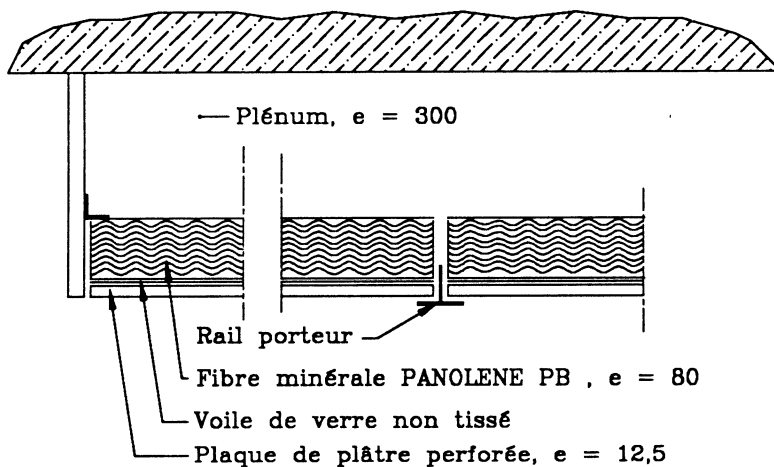
COUPE AA
