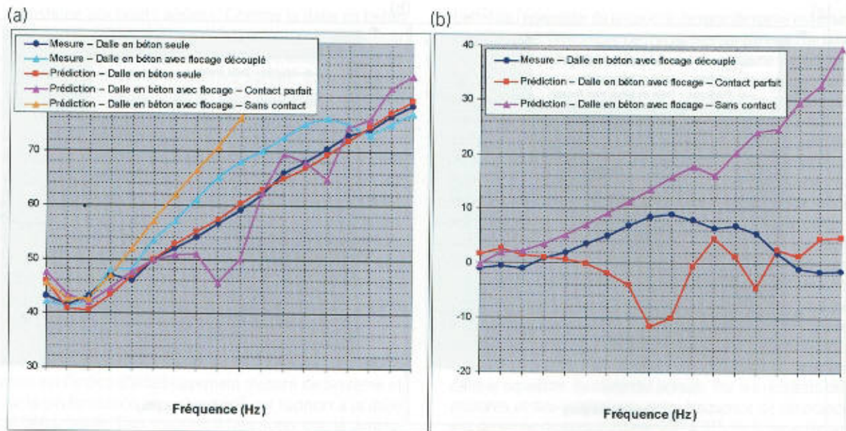
Fig. 6 : Flocage avec système de découplage; (a) indice d'affaiblissement acoustique R et (b) performance acoustique \Delta R
