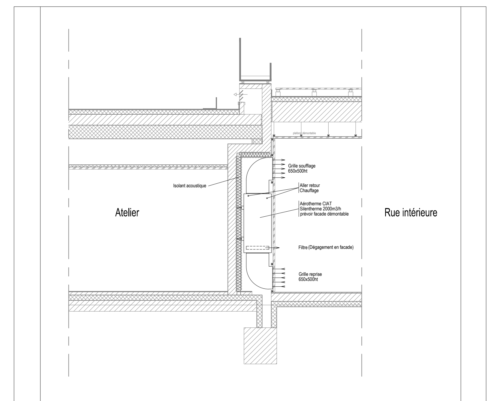
Coupe principe aérothermes
