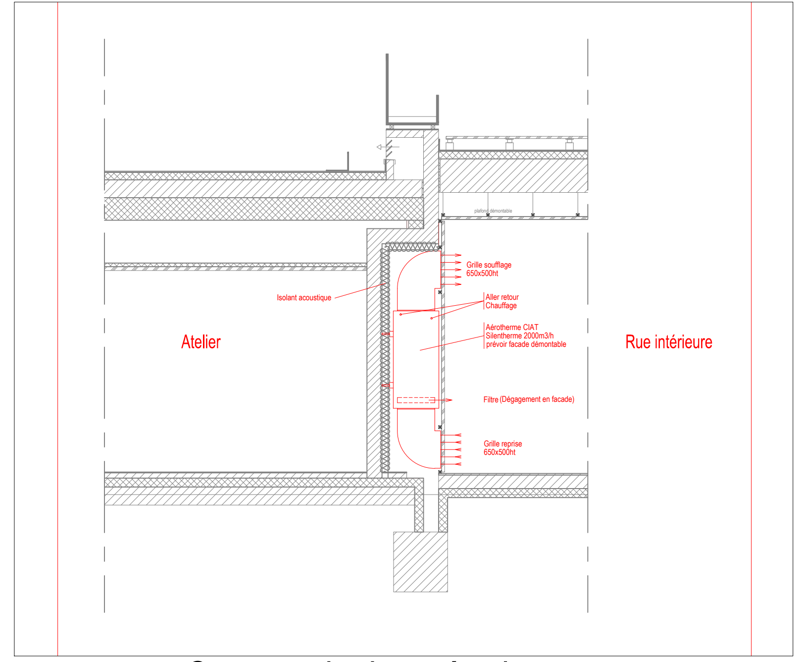
Coupe principe aérothermes
