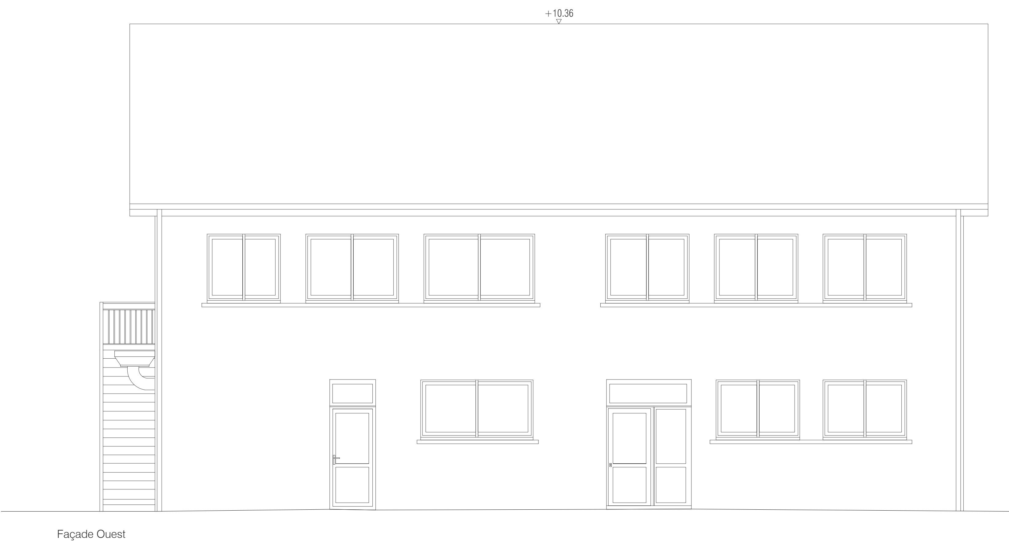
Façade Ouest
