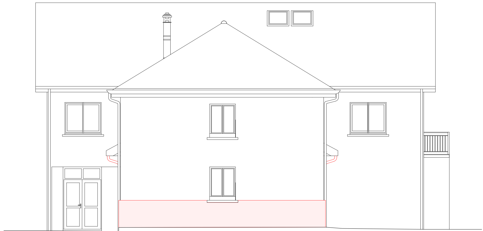
Façade Est
