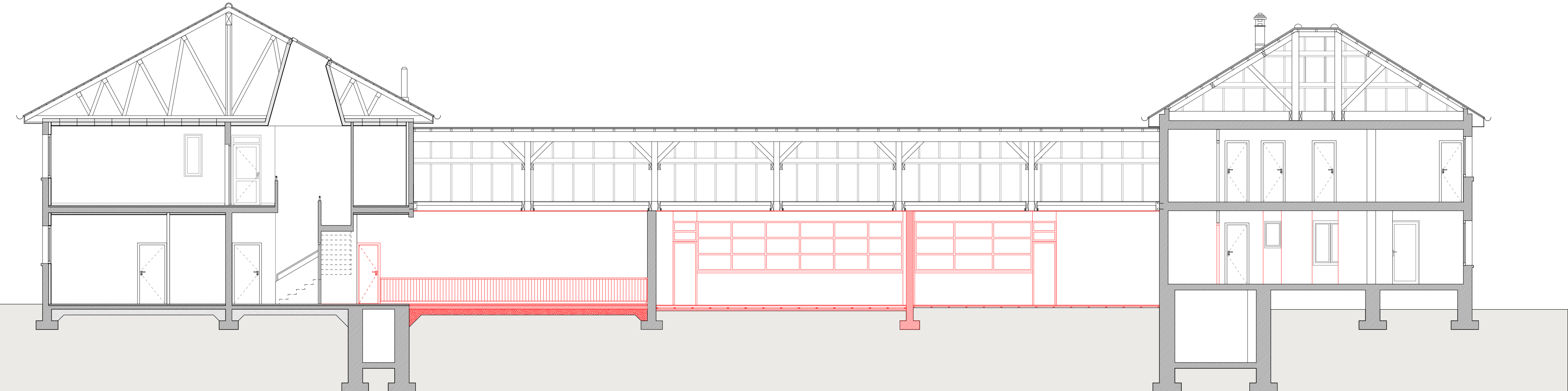
Coupe longitudinale
