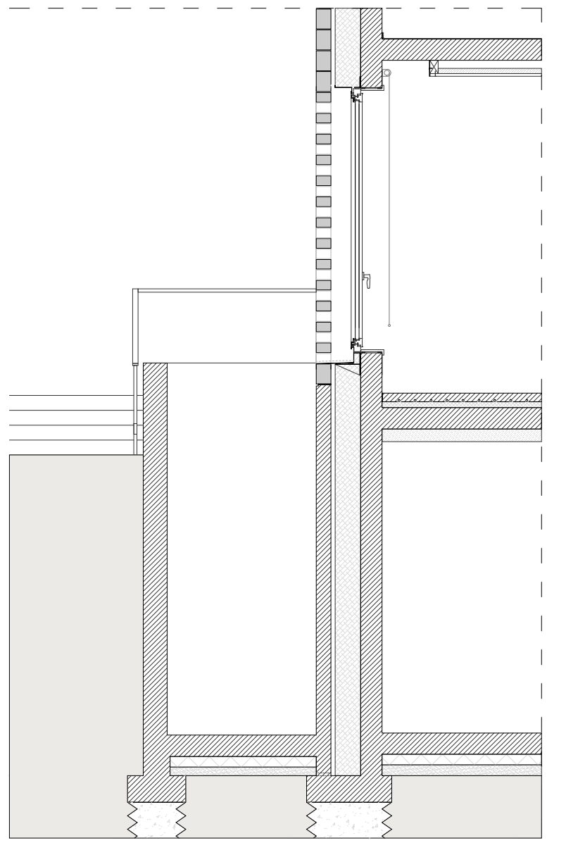
10. Coupe sur l'escalier menant au sous-sol
