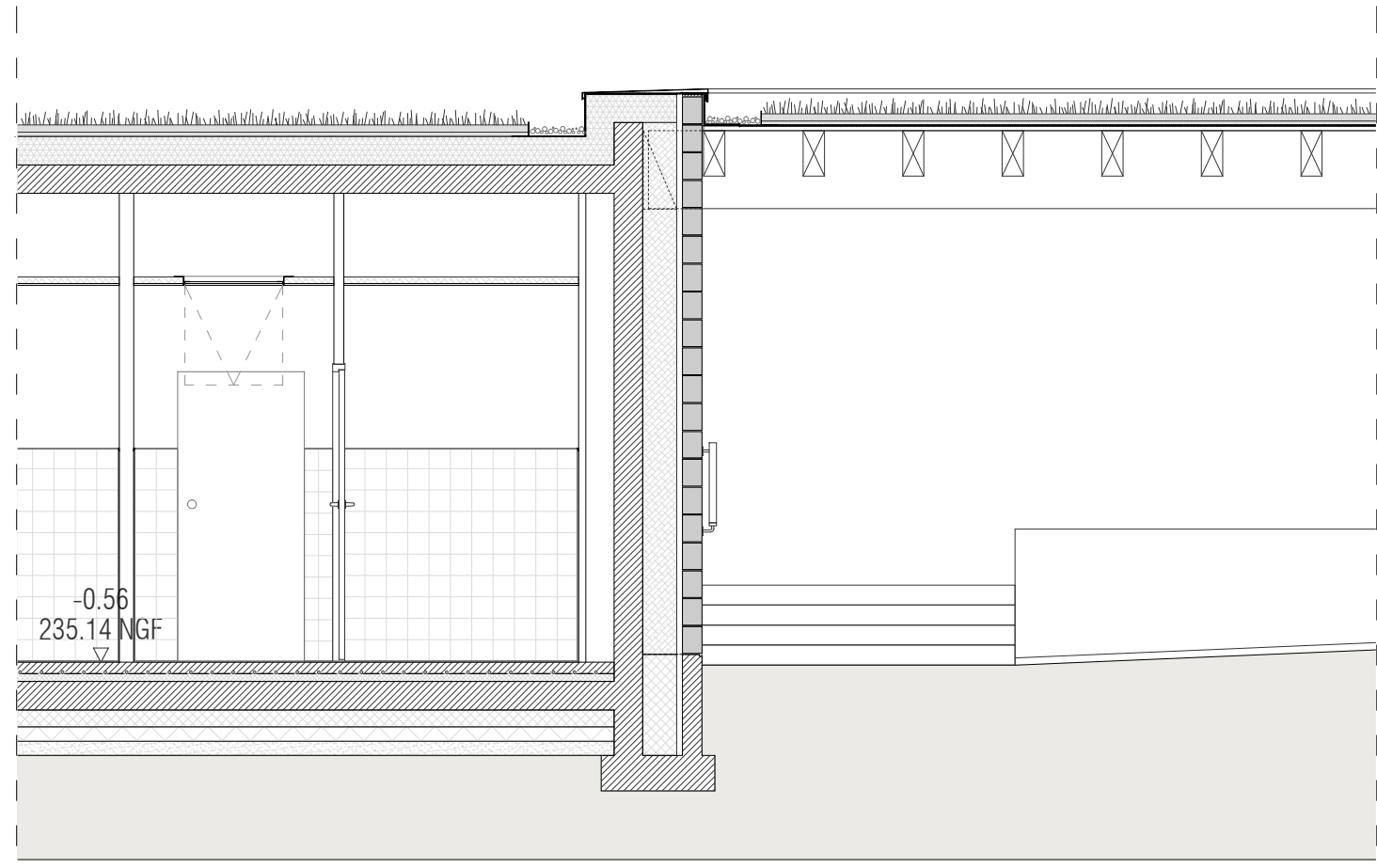
15. Coupe sur le raccord entre le préau et les sanitaires élémentaires
