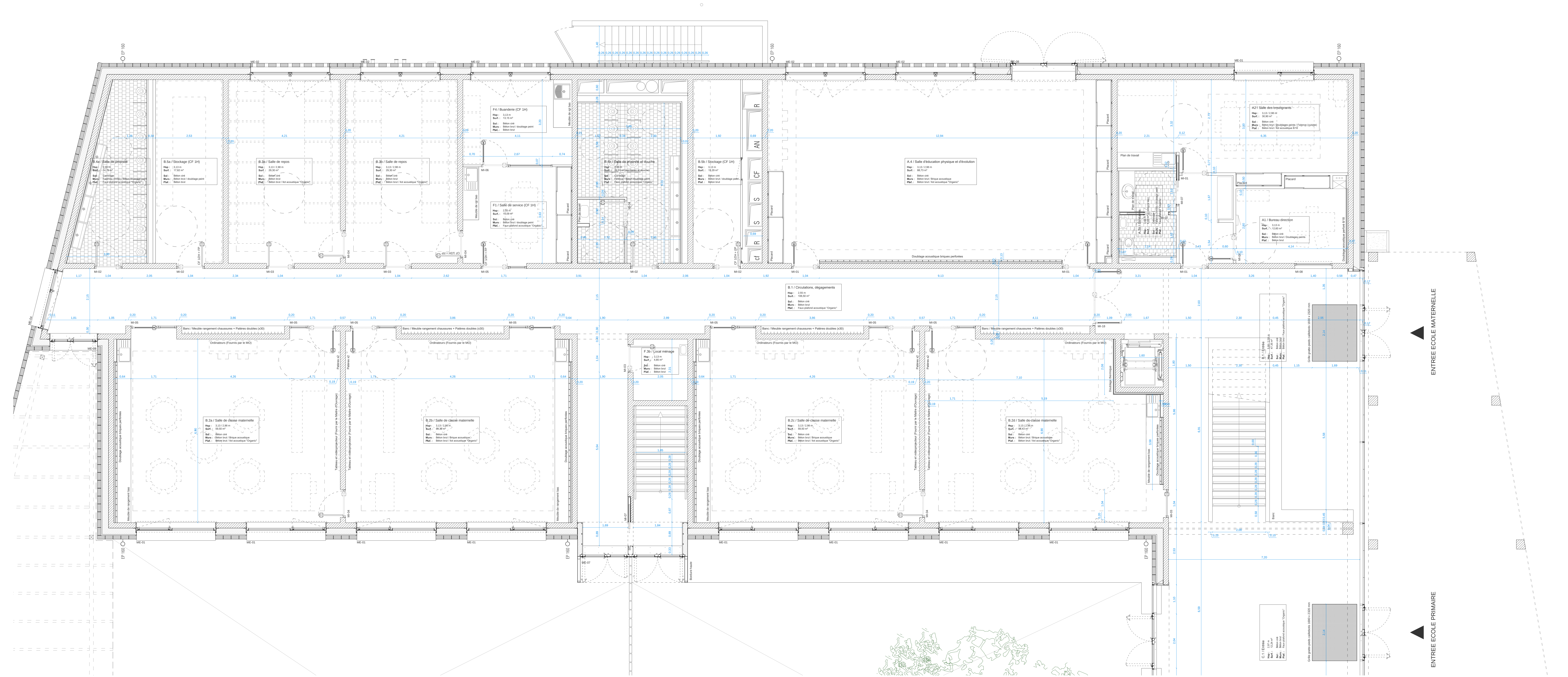
Plan de rez-de-chaussée – Bâtiment école
