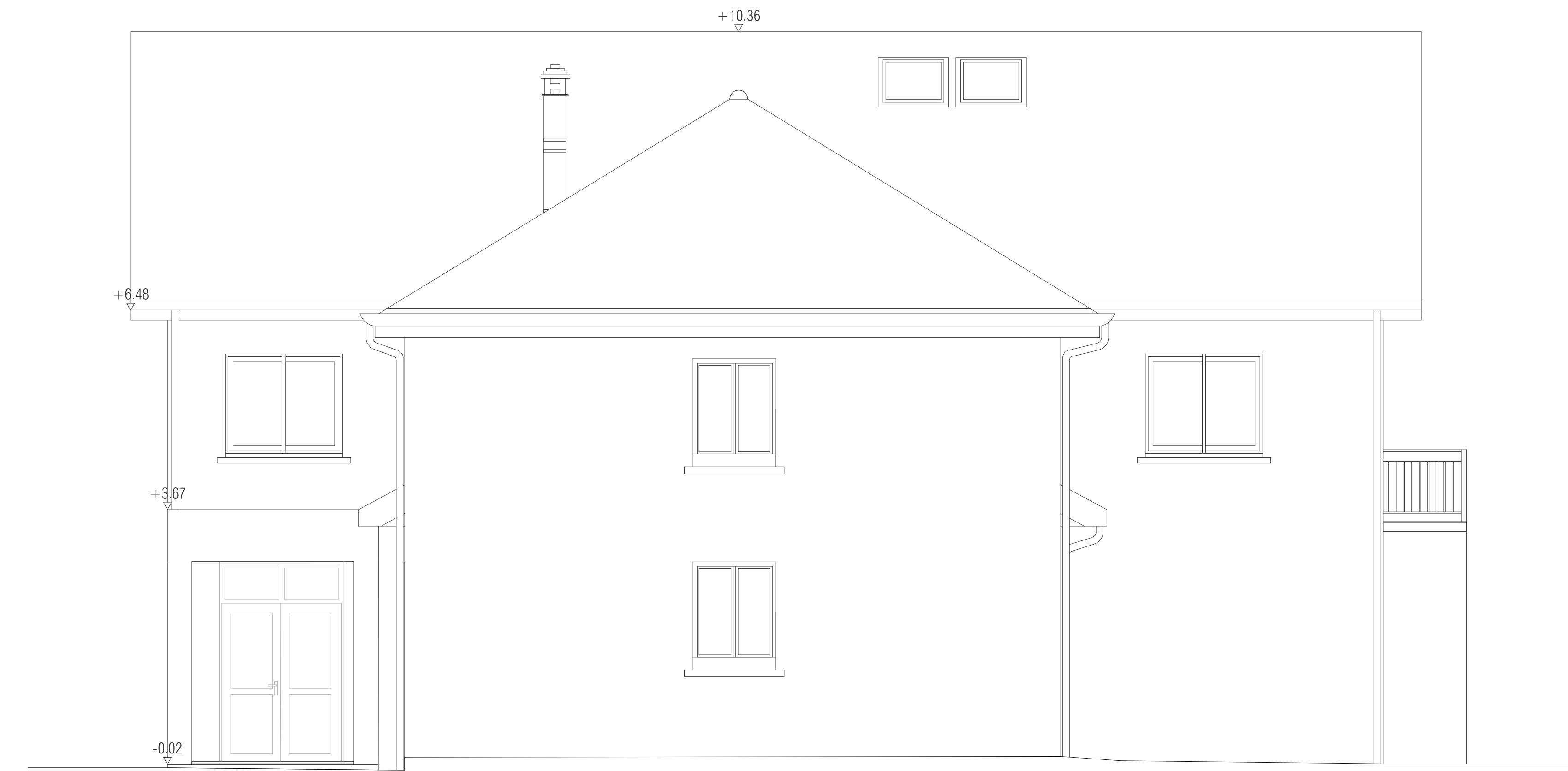
Façade Est
